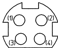
Contact arrangement/端子番号配置図
