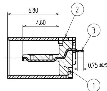
A-A Section / 断面図
