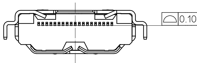
Direction C / C 矢视图
