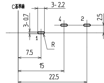
※1.6 参考基板取付孔寸法 (パターン面) (公差 ALL ± 0.1) 数字は端子番号を示す。
