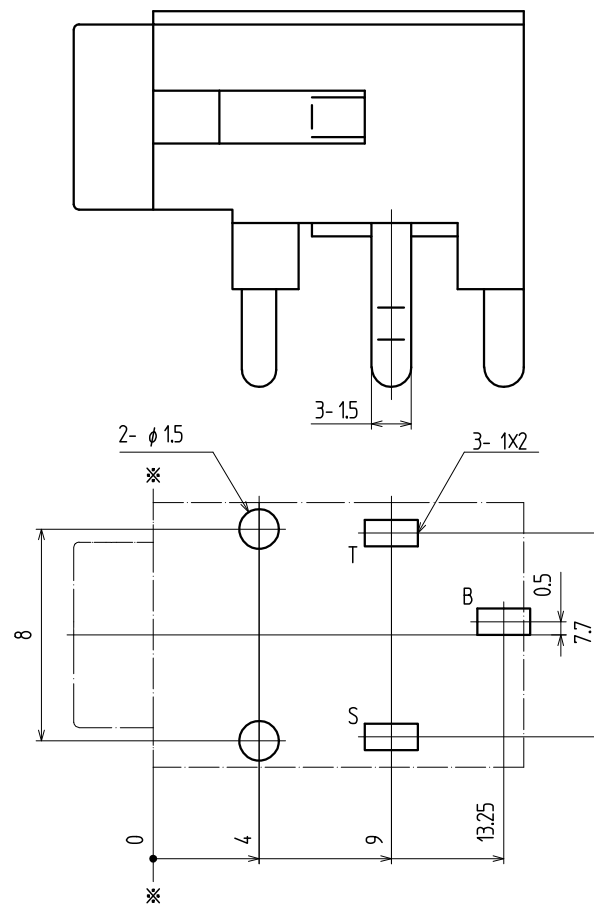
†1.6 参考基板孔寸法図（パターン面より）（公差ALL±0.1）
