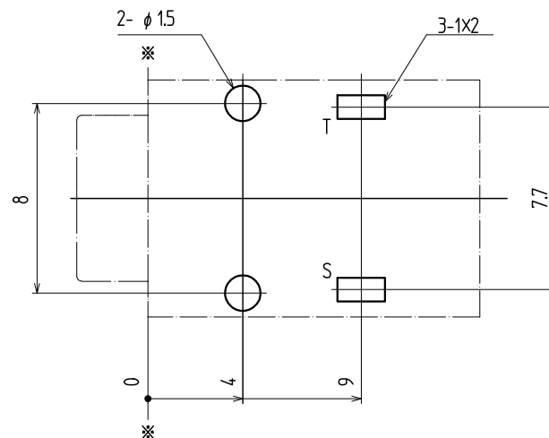
†1.6 参考基板孔寸法図 (パターン面より) (公差ALL±0.1)
