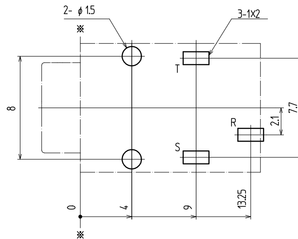
※ 参考基板孔寸法図 (パターン面より) 公差 ALL±0.1
