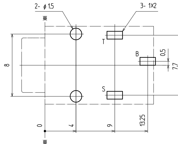
t1.6 参考基板孔寸法図 (パターン面より) 公差 ALL±0.1
