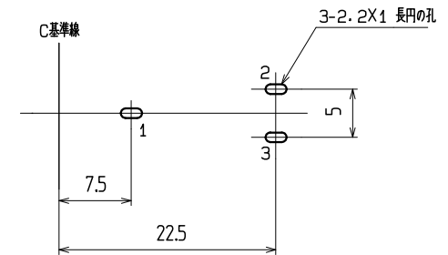
t1.6 参考基板取付孔寸法 (パターン) (公差 ALL \pm 0.1 ) 数字は端子番号を示す。
