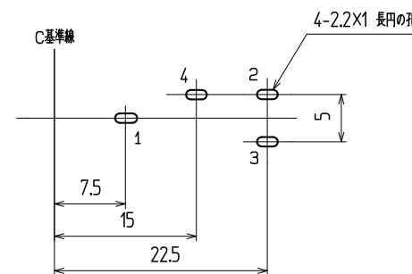
※1.6 参考基板取付孔寸法 (パターン面) (公差 ALL ± 0.1) 数字は端子番号を示す。
