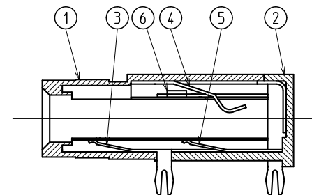
A-A 断面図
