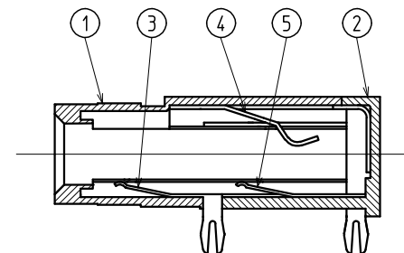
A - A 断面図
