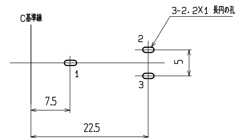
t1.6 参考基板取付孔寸法 (パターン面) (公差 ALL \pm 0.1 ) 数字は端子番号を示す。
