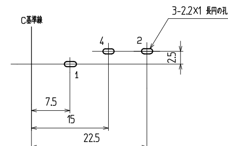
†1.6 参考基板取付孔寸法 (パターン面) (公差ALL \pm 0.1 ) 数字は端子番号を示す。
