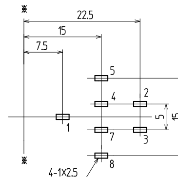
セ1.6 参考基板孔寸法 (パターン面) (公差 ALL ±0.1) (数字は端子番号を示す)
