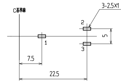
†1.6 参考基板取付穴寸法 (パターン面) (公差 ALL \pm 0.1 ) 数字は端子番号を示す.
