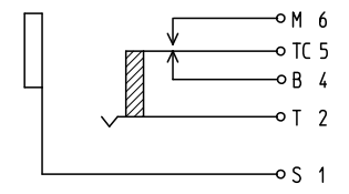
回路図 (数字は端子番号を示す)
