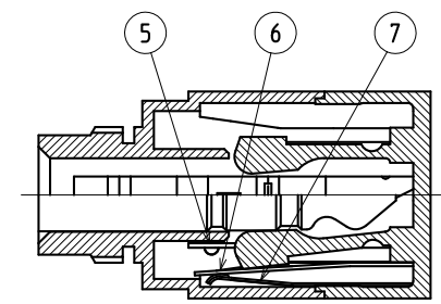
B-B 断面図
