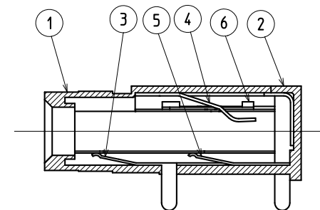
内部構造図
