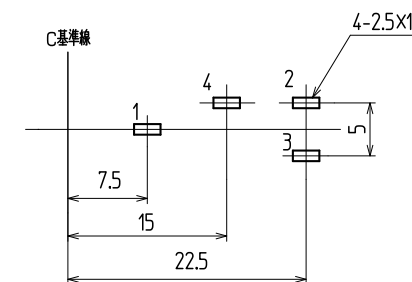
11.6 参考基板取付寸法 (パターン面) (公差 ALL ±0.1) 数字は端子番号を示す。
