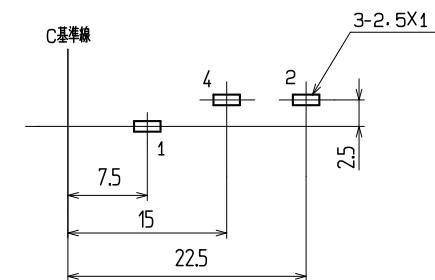
11.6 参考基板取付寸法 (パターン面) (公差 ALL ±0.1) 数字は端子番号を示す。
