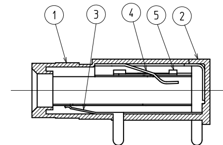
内部構造図
