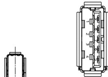
Contact No. layout / コンタクト番号配置図 (Plug insert face) / (プラグ挿入側)
