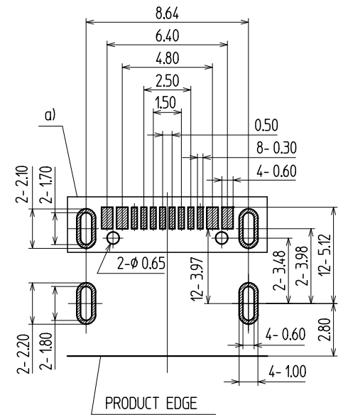
PC BOARD LAYOUT / 参考基板孔寸法図 (Tolerance/公差 ALL±005)
