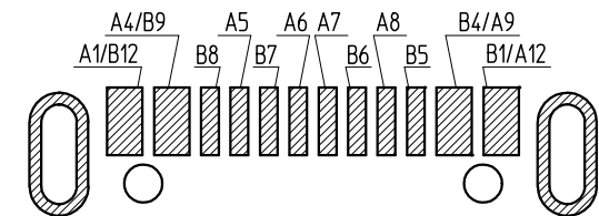
DETAIL OF a) / a) 詳細図
