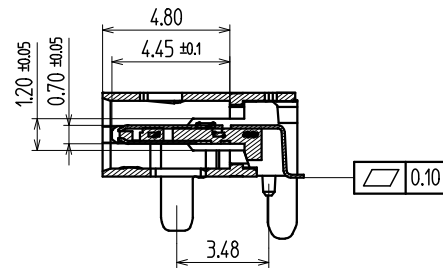
A-A Section / 断面図
