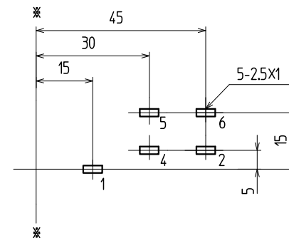
t1.6 参考基板孔寸法 (パターン面) (公差 ALL ±0.1) (数字は端子番号を示す)
