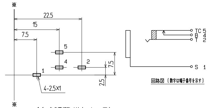
※ 7.1.6 参考基板孔寸法 (パターン面) (公差 ALL ±0.1) (数字は端子番号を示す)
