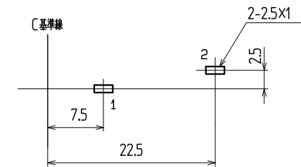
1.6参考基板孔寸法図 (パターン面より) (公差 ALL±0.1) 数字は端子番号を示す。
