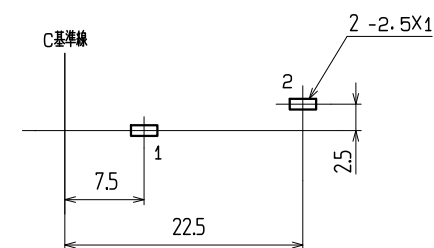
†1.6 参考基板取付寸法 (パターン面)
