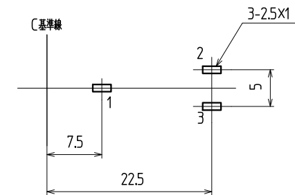
†1.6 参考基板取付寸法 (パターン面)
