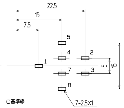
基準線 C 7-2.5X1 ±1.6 参考基板孔寸法 (パターン面) (公差 ALL ±0.1) (数字は端子番号を示す)
