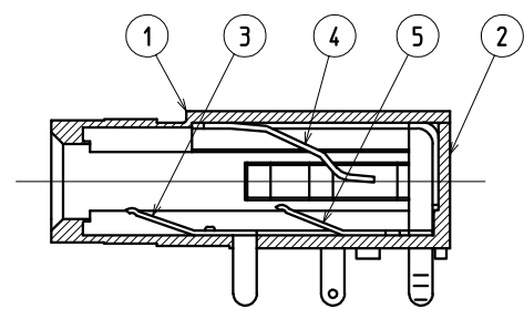
A-A断面図
