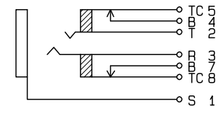
回路図 (数字は端子番号を示す)
