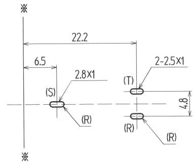
参考基板孔寸法 (半田面よ見る) (公差 ALL±0.1)
