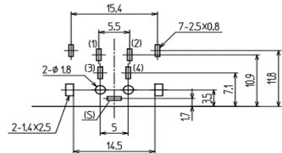
Dimensions of PC board holes / 参考基板孔 Parts side view / 部品面より見る
