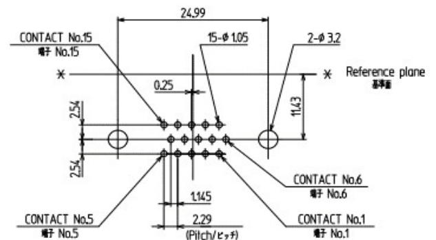
Dimensions of PC board holes/参考基板孔寸法 (Printed-side view, Tolerance all±0.1)/パターン側より見る 公差±0.1
