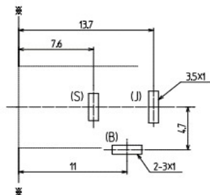
Dimensions of PC board holes / 参考基板孔 Tolerance / 公差 ALL+0.1 Parts-side view / 部品面側より見る
