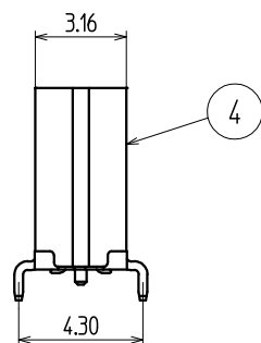
A-A Sec / 断面図
