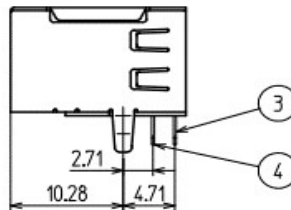
Front edge of connector コネクタフロントエッジ
