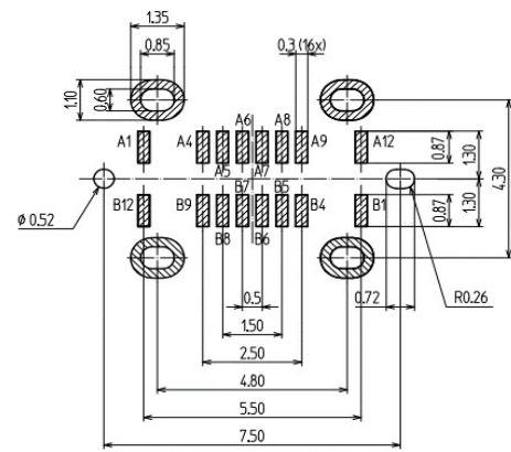
PC BOARD LAYOUT / 参考基板寸法図 (S=10/1) (Tolerance/公差 ALL±0.05)(Parts Side/部品面)
