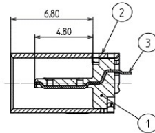
A-A Section / 断面図
