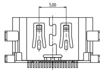
Direction B / B 矢視図
