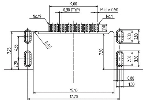
Dimensions of P.C.B layout 参考基板寸法図 (t=1.0~1.2)
