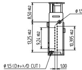
B 矢視図
