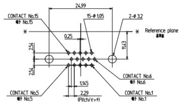
Dimensions of PC board holes / 参考基板孔寸法図 (Printed-side view, Tolerance all±0.1) / (バタ-ン側より見る 公差±0.1)
