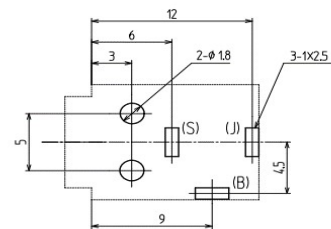
Dimensions of PC board holes / 参考基板孔 Parts side view / 部品面より見る
