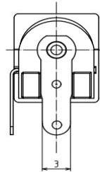
※ Dimensions of PC board holes / 参考基板孔 Parts side view / 部品面より見る
