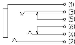
CIRCUIT DIAGRAM / 回路図
