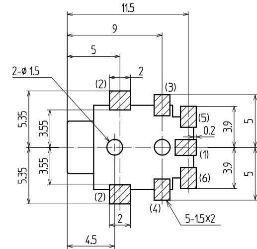
PC BOARD LAYOUT / 参考基板孔寸法図 (Tolerance/公差 ALL±0.1)(Parts Side/部品面)
