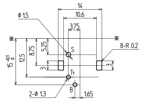
Referential Dimensions of PC board holes / 参考基板孔寸法図 (Tolerance / 公差 ALL±0.1/Printed-side view / パターン側) M1.6
