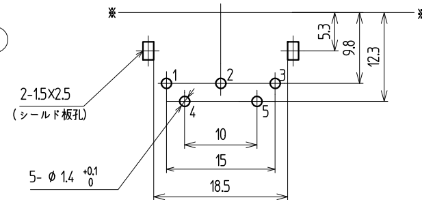
参考基板寸法図 (パターン側) 公差ALL±0.1
