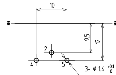
参考基板穴寸法図 (パターン側) 公差 ALL ± 0.1
