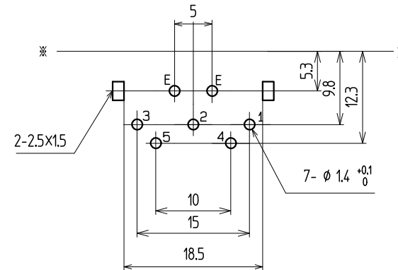
t1.6 参考基板穴寸法図 (パターン側) 公差 ALL ± 0.1
