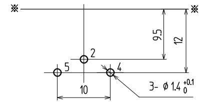
†1.6 参考基板孔寸法図 (パターン側)(公差all±0.1)
