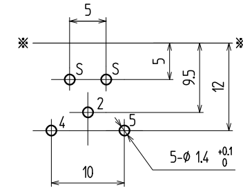
t1.6 参考基板孔寸法図 (パターン側)(公差all±0.1)
