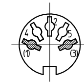
ピン配列 (プラグ挿入側)
