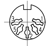
ピン配値図 (プラグ挿入側)
