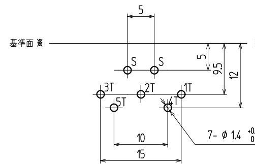
t1.6 参考基板孔図
