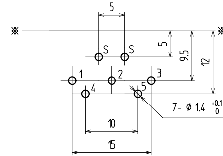
†1.6 参考基板孔寸法図 (パターン側)(公差all±0.1)
