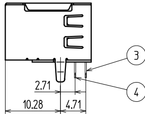
Front edge of connector コネクタフロントエッジ
