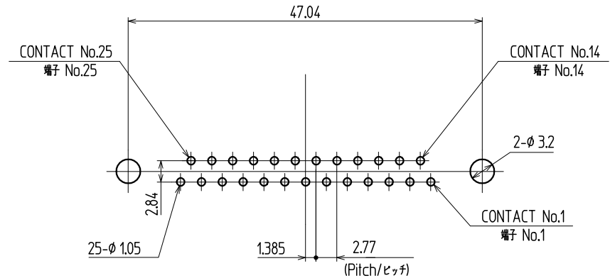
Dimensions of PC board holes / 参考基板孔寸法図 (Printed-side view, Tolerance all ±0.1) / (パターン側より見る 公差 ±0.1)
