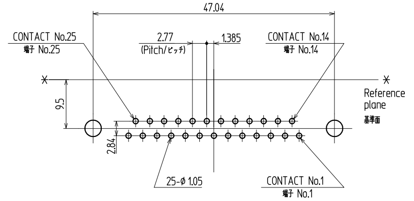
Dimensions of PC board holes / 参考基板孔寸法図 (Printed-side view, Tolerance all ±0.1) / (バタ-ソ側より見る 公差±0.1)
