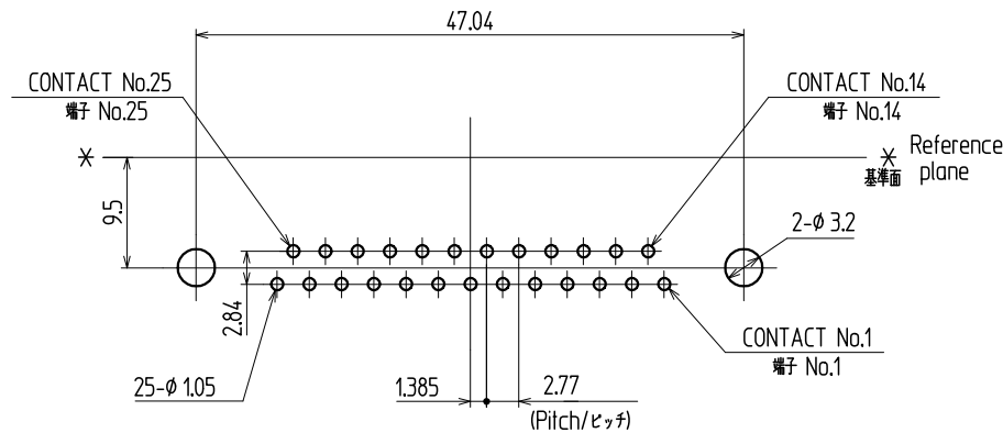
Dimensions of PC board holes / 参考基板孔寸法図 (Printed-side view, Tolerance all ±0.1) / (パターン側より見る 公差±0.1)
