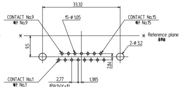
Dimensions of PC board holes / 参考基板孔寸法 (Printed-side view, Tolerance all ±0.1) / (プリント側より見る 公差±0.1)
